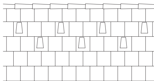
23. Két sorban minden harmadik cserép szellőzőcserép – Granite 2,20 db szellőzőcserép / fm (kb. 35 cm 2 / fm kiszellőzés)
