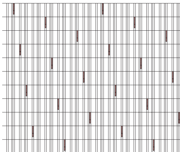
25. Minden hetedik cserépbe akasztott hófogó (kb. 1,4–1,5 db / m 2 )
