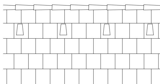
21. Minden harmadik cserép szellőzőcserép – Granite 1,10 db szellőzőcserép / fm (kb. 18 cm 2 / fm kiszellőzés)
