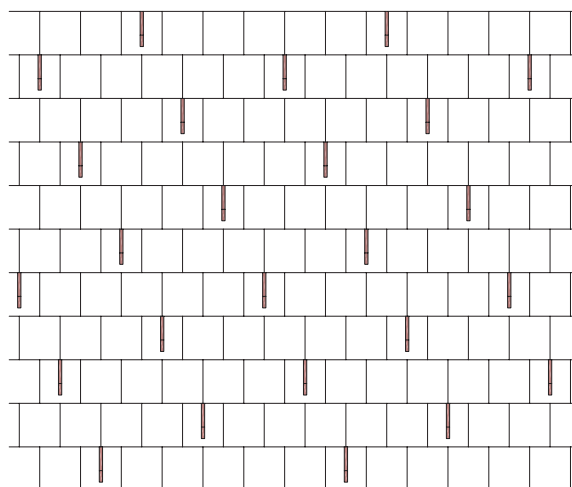
28. Minden hatodik cserépbe akasztott hófogó (kb. 1,7–1,8 db / m 2 )
