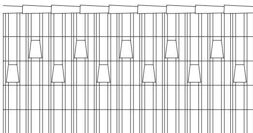
20. Két sorban minden második cserép szellőzőcserép – Toscana 3,33 db szellőzőcserép / fm (kb. 47 cm 2 / fm kiszellőzés)
