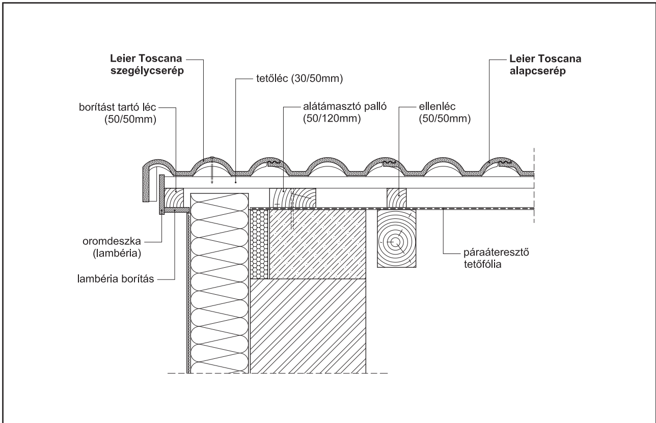
5/12 Ormszegély részlet Leier Toscana 1:10
