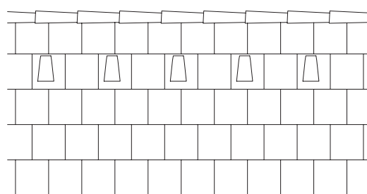
22. Minden második cserép szellőzőcserép – Granite 1,64 db szellőzőcserép / fm (kb. 26 cm 2 / fm kiszellőzés)
