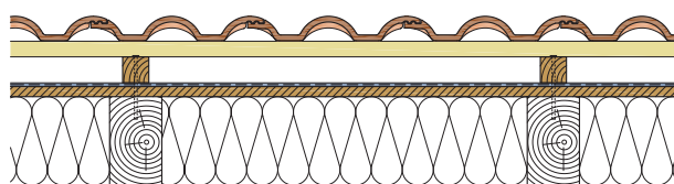
2. Aljazaton fekvő alátét fedés
