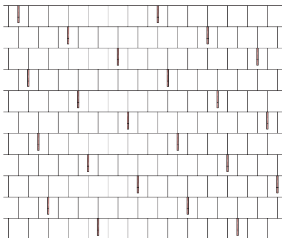
27. Minden hetedik cserépbe akasztott hófogó (kb. 1,4–1,5 db / m 2 )
