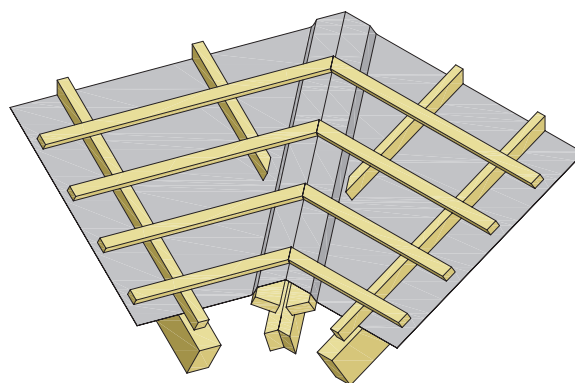
5. Alátét héjazat vápánál
