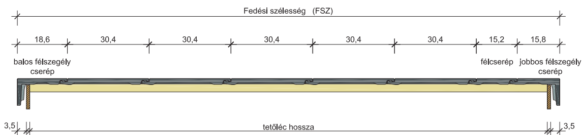
9. Fedési szélesség – Granite
