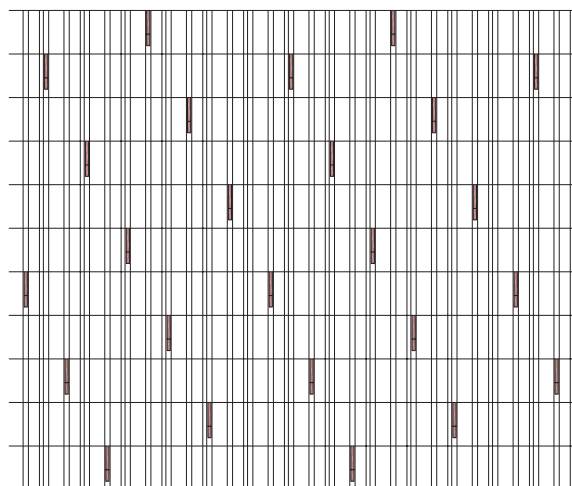
26. Minden hatodik cserépbe akasztott hófogó (kb. 1,7–1,8 db / m 2 )
