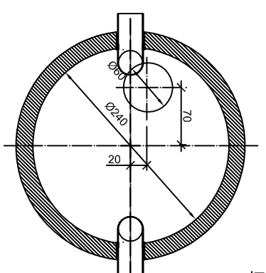
Keretszmetszet
