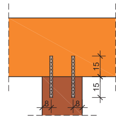
19. Bekötőszalag helye
