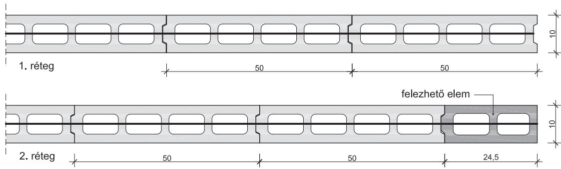
23. Falvég: Leier beton válaszfalelem VF 10
