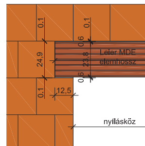
42. Méretek – Leier MDE nyílásáthidaló
