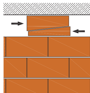
5. Válaszfal kiékelése
