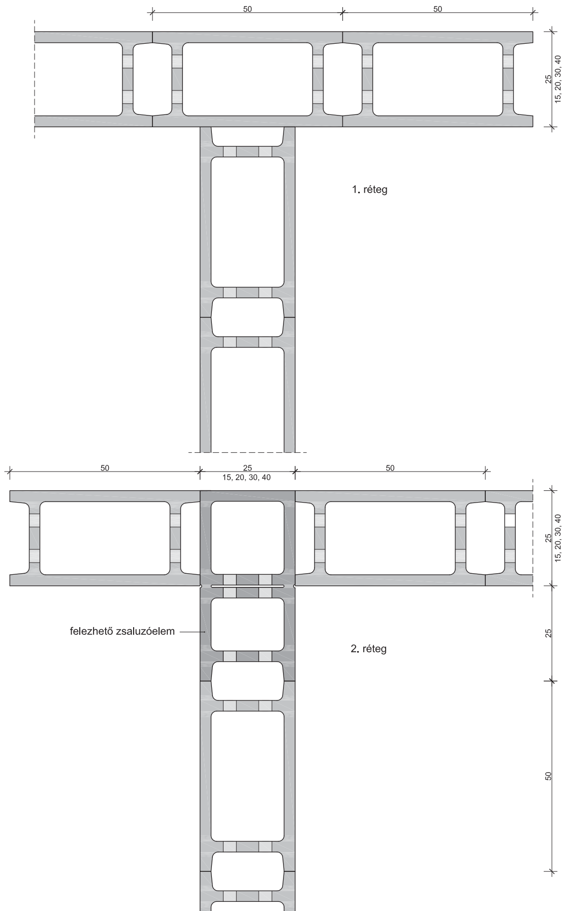
26. Falcsatlakozás: Leier beton zsaluzóelem (ZS 15, ZS 20, ZS 25, ZS 30, ZS 40)
