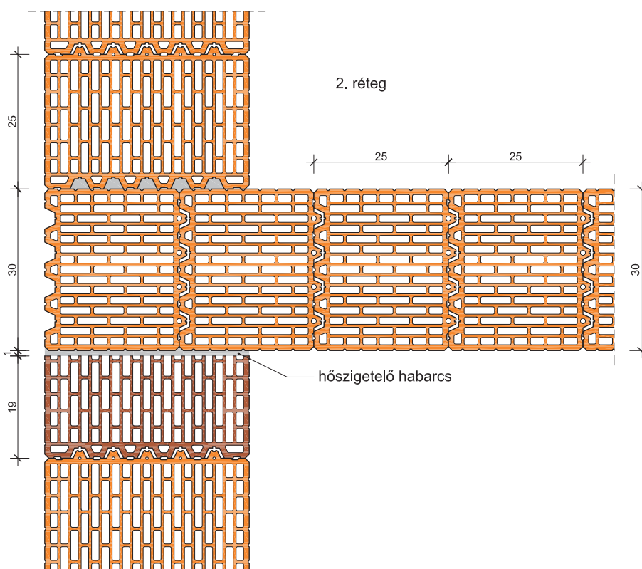
72. Falcsatlakozás: LeierPLAN 38 Pro – LeierPLAN 30 Pro / LeierPLAN 38 N+F – LeierPLAN 30 N+F Leiertherm 38 Pro – Leiertherm 30 Pro / Leiertherm 38 N+F – Leiertherm 30 N+F
