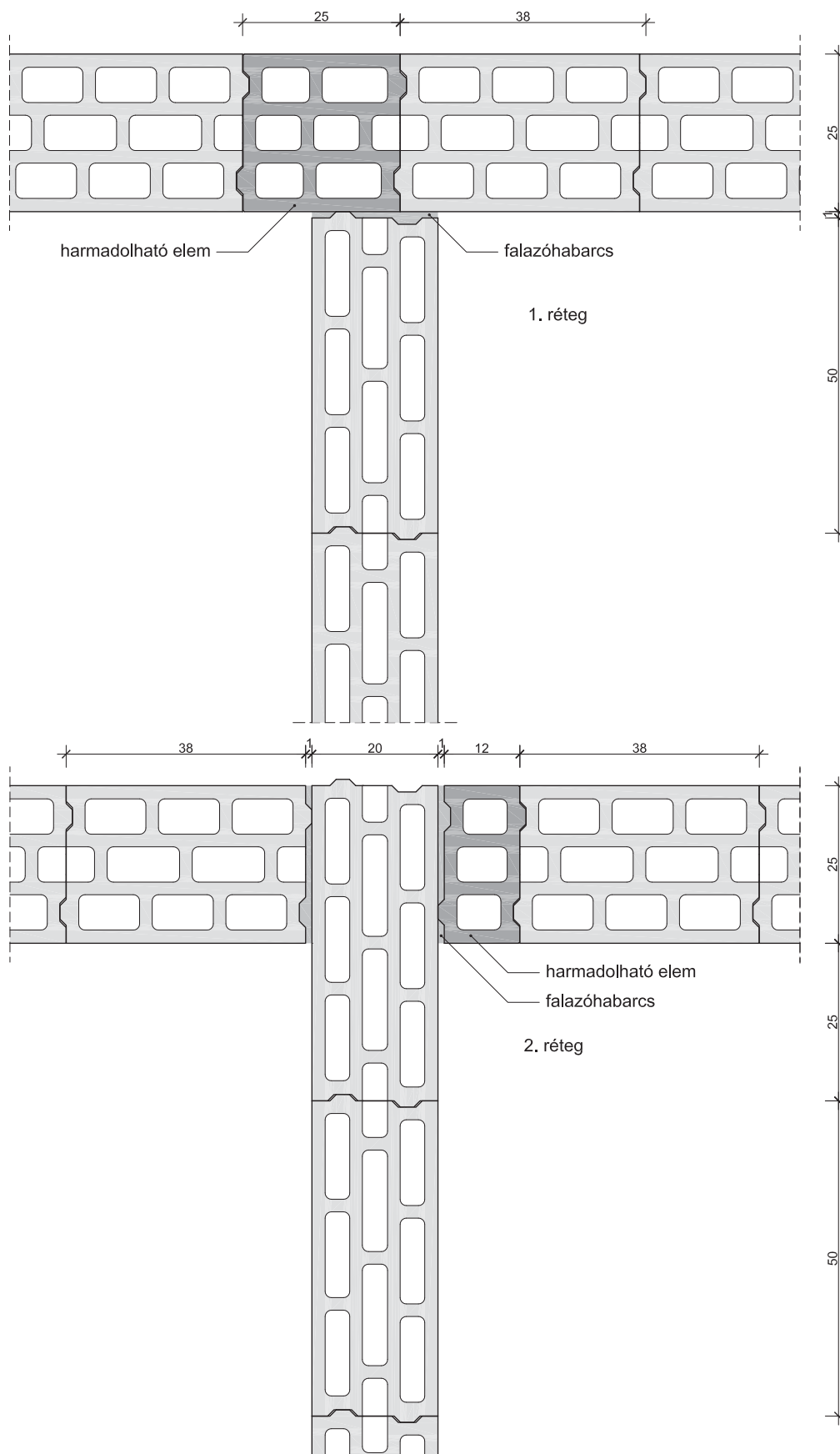
19. Falcsatlakozás: Leier beton főfalelem FF 25 – Leier beton főfalelem FF 20
