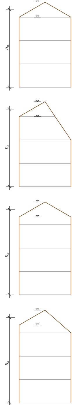
1. Építménymagasság értelmezése
