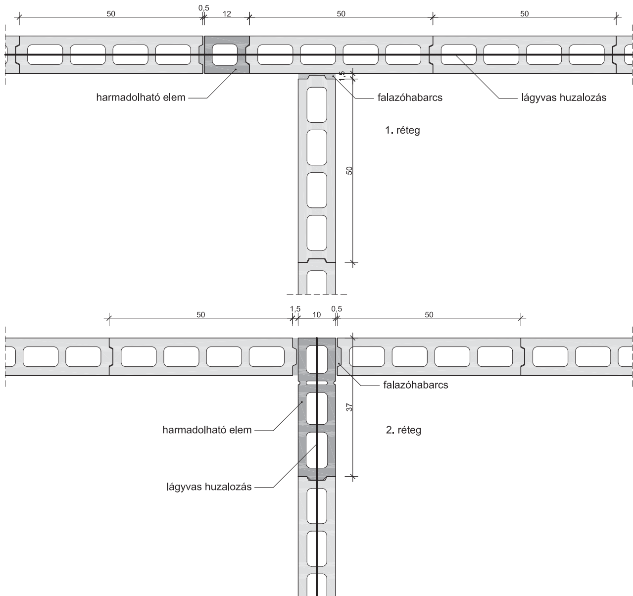
24. Falsarok: Leier beton válaszfalelem VF 10
