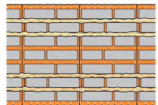
12. LeierFIX univerzális építési ragasztó felhordása különböző falazóelemekre
