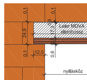
45. Méretek – Leier MDA és Leier MDVA nyílásáthidaló
