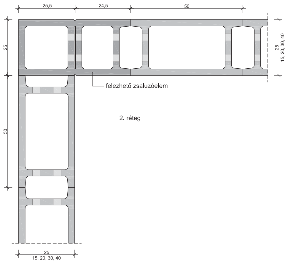
25. Falsarok: Leier beton zsaluzóelem (ZS 15, ZS 20, ZS 25, ZS 30, ZS 40)
