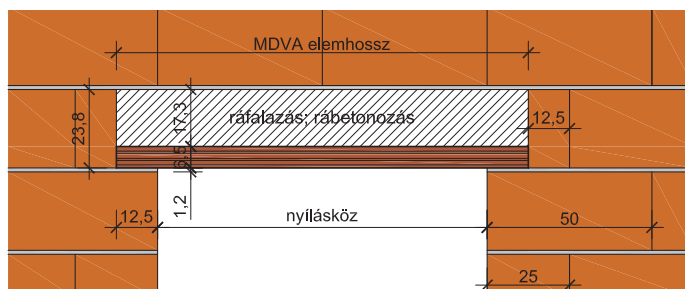
16. Leier MDVA nyílásáthidaló oldalnézet
