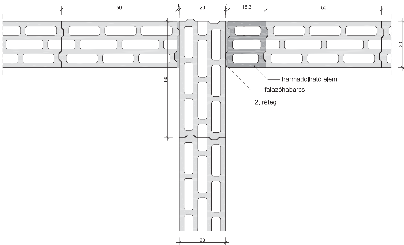
21. Falcsatlakozás: Leier beton főfalelem FF 20
